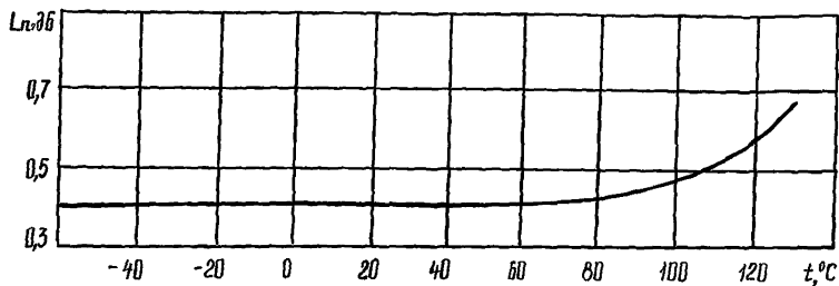
Характеристика потерь запирающего в зависимости от температуры среды
