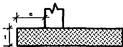
Тип 1. Армирование стальной фиброй
