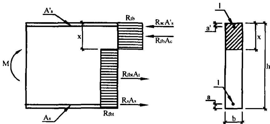
Рис.3. Схема усилий и эпюра напряжений в сечениях, нормальных к продольной оси изгибаемого железобетонного элемента прямоугольного сечения при комбинированном армировании 1 - стержневая или проволочная арматура
