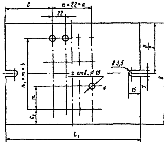
Развертка
