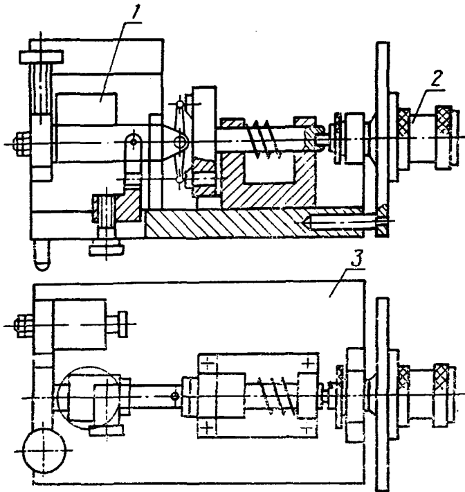
1—индикатор; 2—микрометрическая головка; 3—плата
