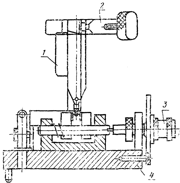
1—индикатор; 2—зажимы; 3—микрометрическая головка; 4—плита
