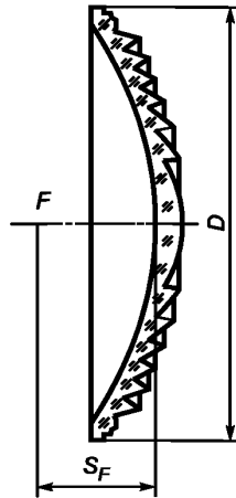
Рисунок 5 — Светофильтр-линза СЛ 139
