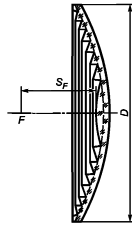
Рисунок 6 — Линза ступенчатая ЛС 212 и ЛС 160
