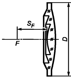
Рисунок 4 — Светофильтр-линза СЛ 70 или линза ступенчатая ЛС 70
