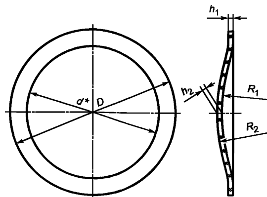
Рисунок 2 — Светофильтр вогнуто-выпуклый типа СВВ
