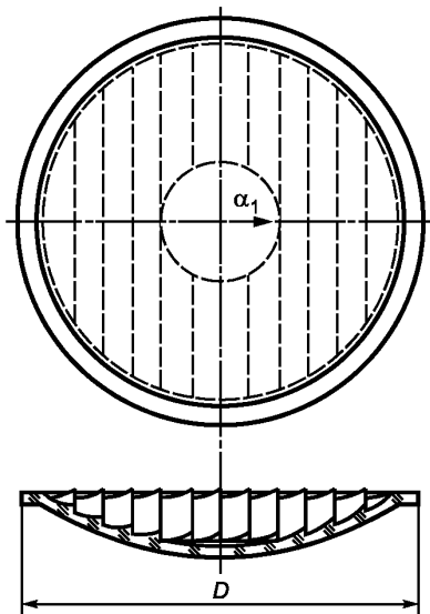
Рисунок 7 — Односторонний рассеиватель
