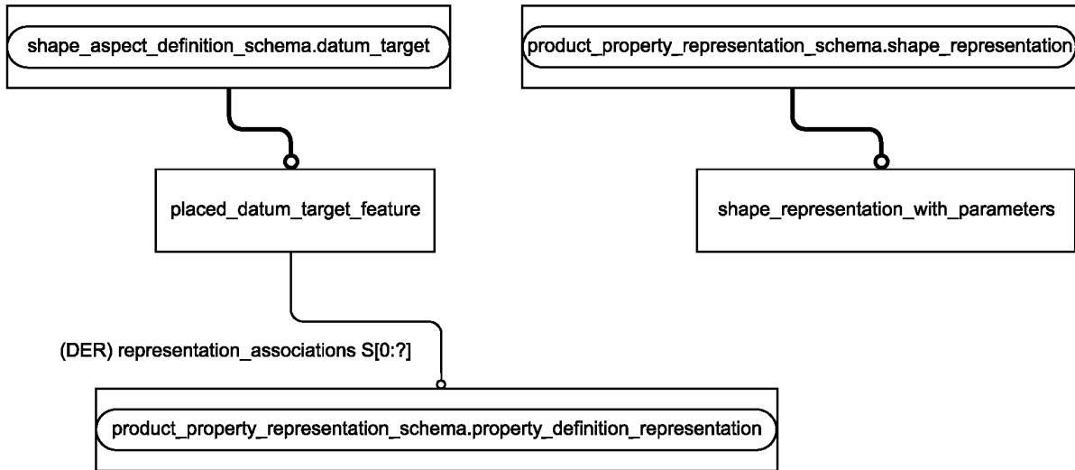
Рисунок D.2 — Представление ИММ на уровне объектов в формате EXPRESS-G
