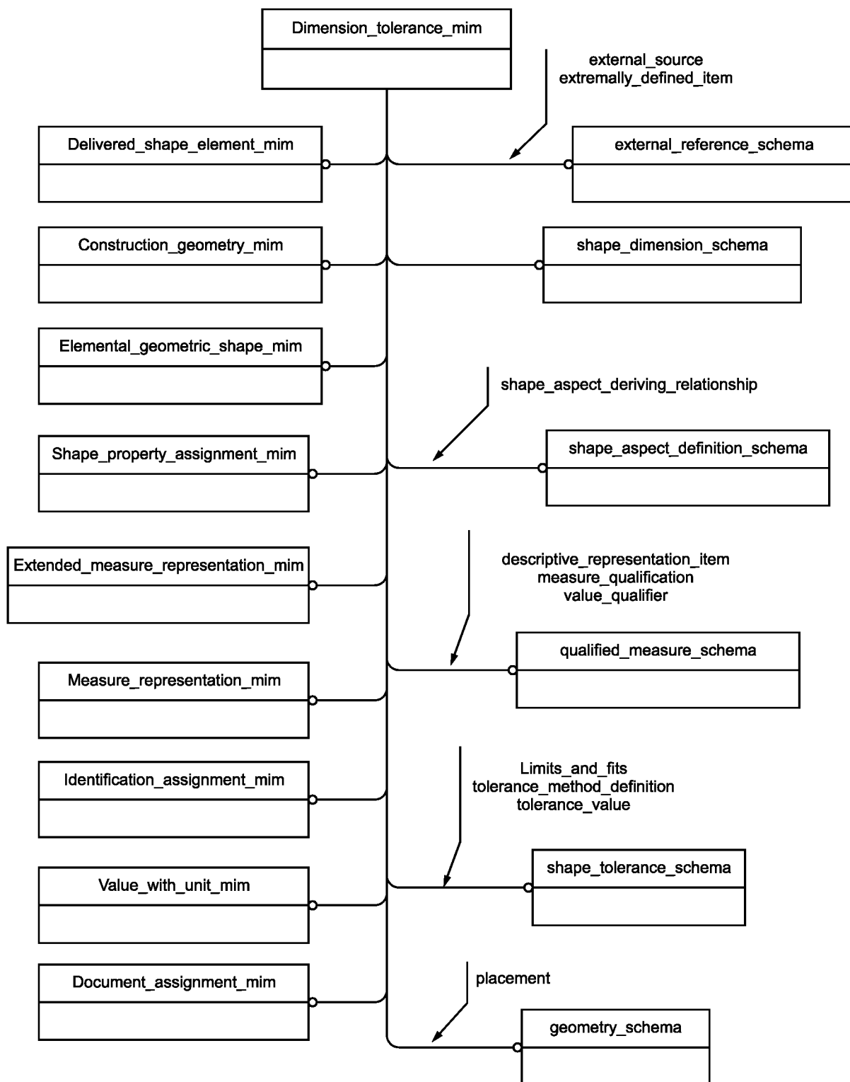
Рисунок D.1 — Представление ИММ на уровне схем в формате EXPRESS-G
