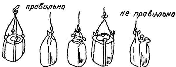
Рис. 5. Стропление контейнеров: а) типа МК-И; б) типа МКР и МКО-С; в) типа МКР-М
