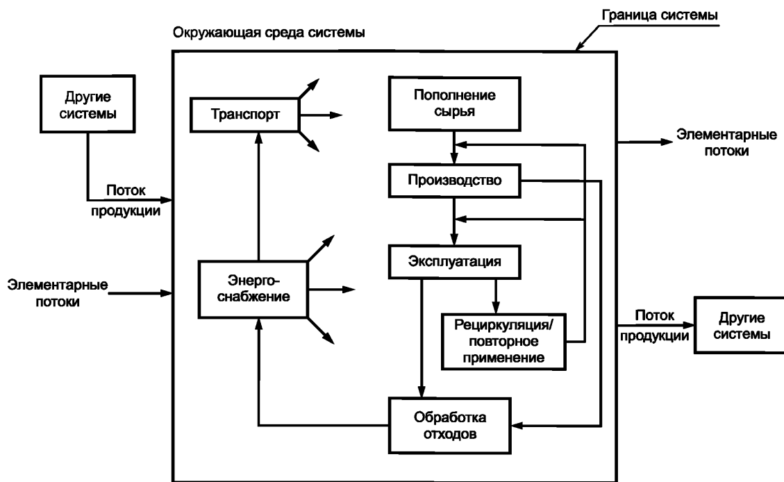
Рисунок 2 — Пример производственной системы для ОЖЦ
