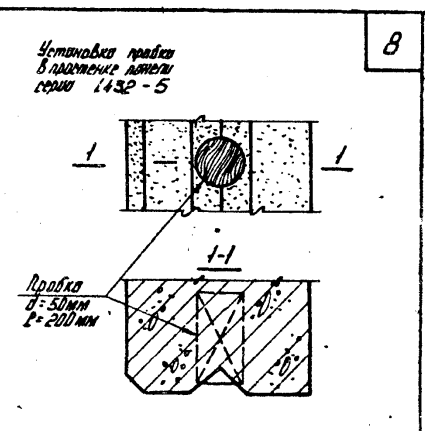
Установка пробок в проемы латки серии 1432-5
