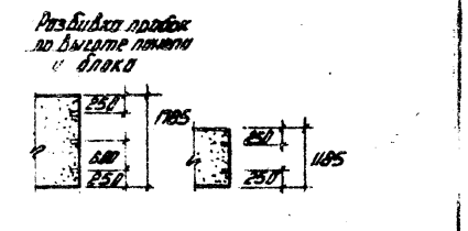
Разбивка пробок по высоте латки и стекла
