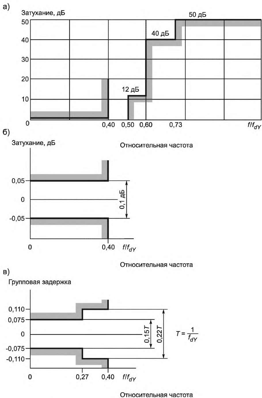
Рисунок 4 — Характеристики фильтров низких частот для сигналов яркости E_{\gamma}
