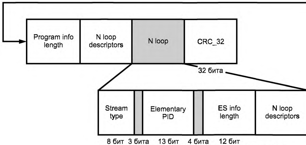
Рисунок А.6 — Диаграмма полей секций таблицы PMT
