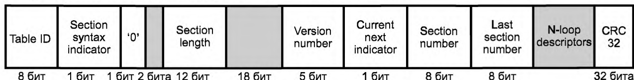
Рисунок А.5 — Диаграмма полей секции таблицы CAT
