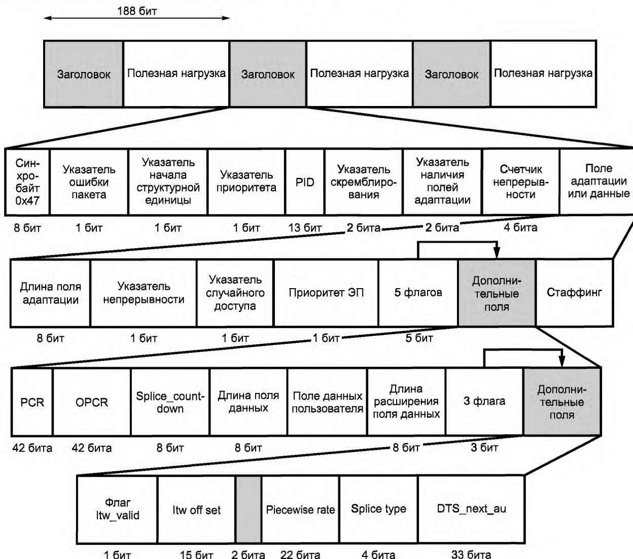
Рисунок А.2 — Структура основных полей транспортного потока MPEG
