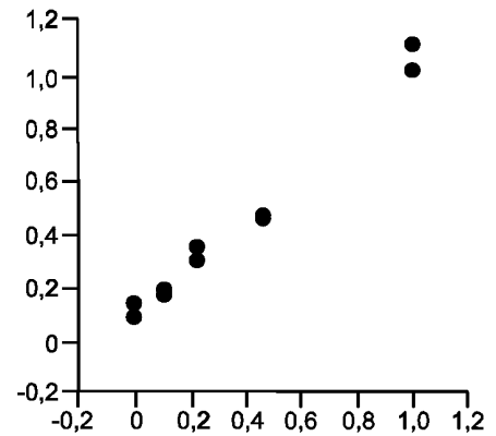
Рисунок N.4 — Для использования с удлинённой шкалой, только если SD (среднеквадратическое отклонение) возрастает с ростом y
