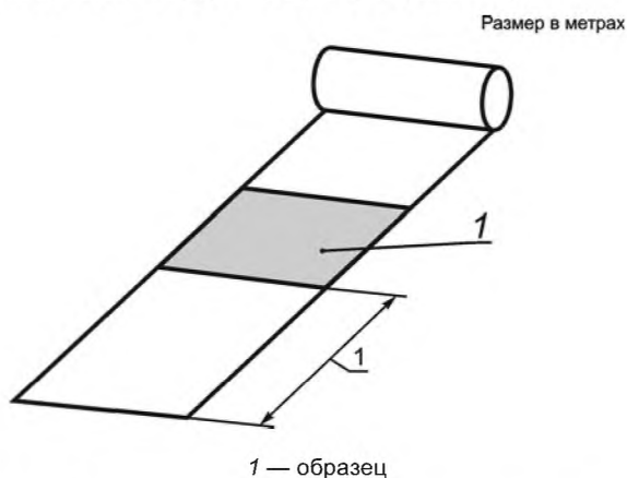
Рисунок А.1 — Схема отбора образца твердого материала из рулонов
