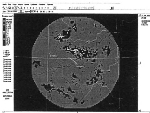
Рисунок А.2. Пример отображения информации об осадках, полученной от автоматизированного метеорологического радиолокационного комплекса
