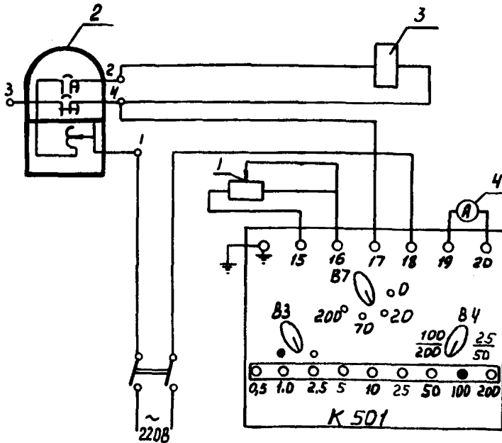
Рис.6. Схема проверки коммутационной способности контактов реле от устройства УИЗ-1: 1 - проволочный реостат 300 Ом, 2 А; 2 - реле; 3 - электромагнит отключения; 4 - внешний амперметр 5 А, класс точности I,0-I,5
