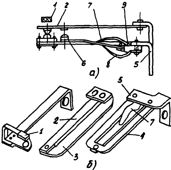
Рис.2. Контактная система реле РТ-85, РТ-86 и РТ-95:
