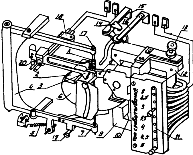
Рис.1. Кинематическая схема реле:
