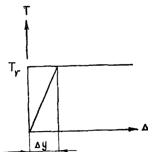
Рис. 1. Расчетная схема отсеков при замыкании деформационного шва:
