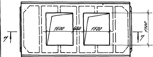
Рис. 4. Плита для железобетонных сборных конструкций
