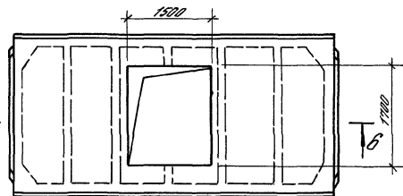
Рис. 3. Плита с проемом в планке \phi 1000 или 1450 мм для пропускки вентилятора
