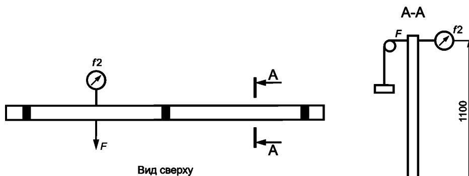
Рисунок 11 — Схема испытания поручней
