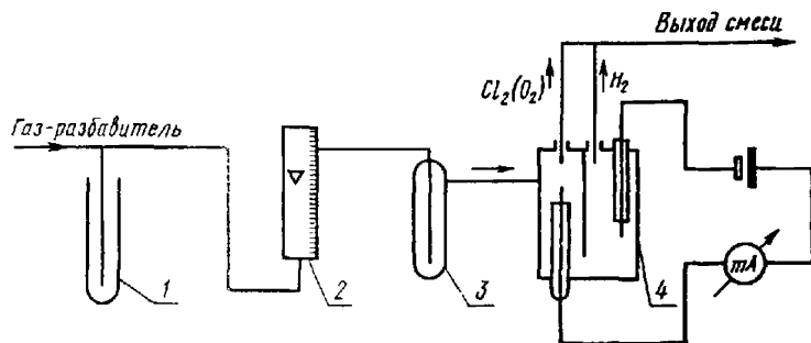
1—маностат; 2—измеритель расхода; 3—увлажнитель; 4—электролизер.
