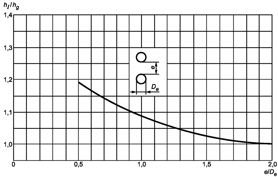
Рисунок 3 — Значения h_l/h_g для двух кабелей, расположенных в вертикальной плоскости
