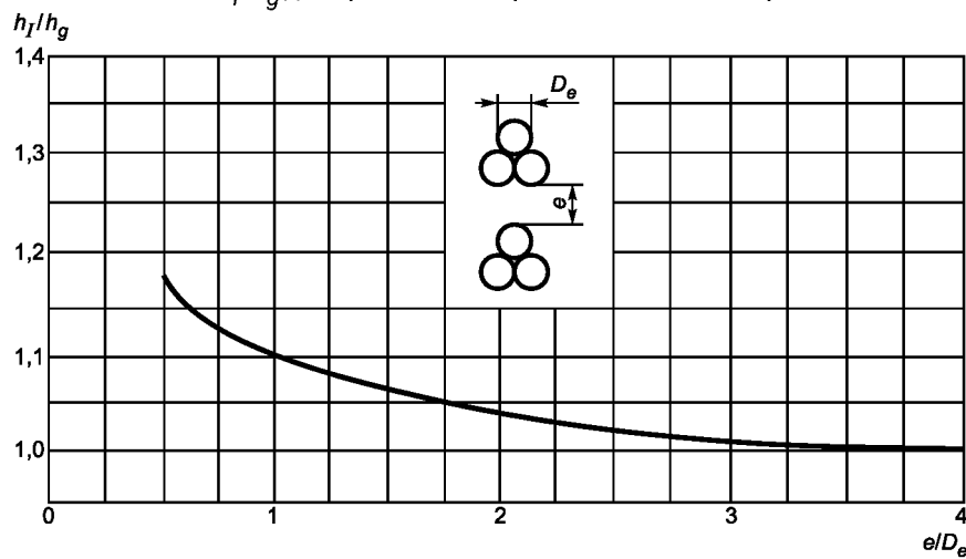
Рисунок 5 — Значения h_l/h_g для двух групп из трех кабелей, расположенных треугольником, в вертикальной плоскости
