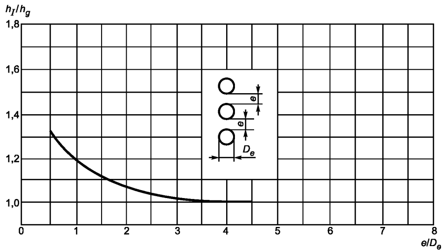
Рисунок 4 — Значения h_l/h_g для трех кабелей, расположенных в вертикальной плоскости
