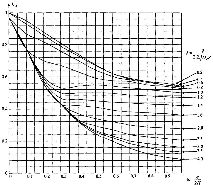
Рис. п.4.6. Графики для определения коэффициента C_p
