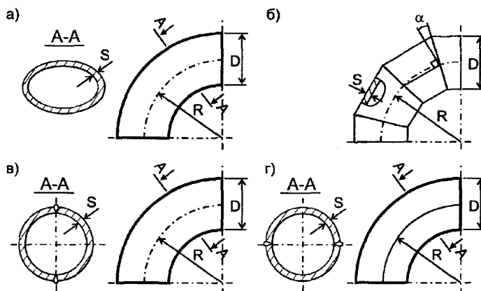
Рис. 3.1. Отводы: а - гнутый; б - секторный; в, г - штамповарной
