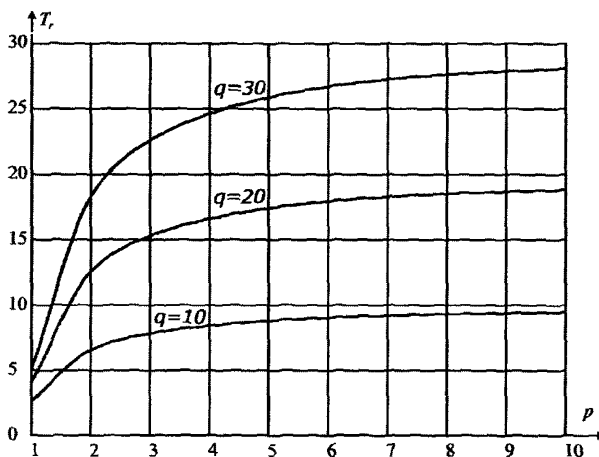
Рис. п.б.1. К определению назначенного ресурса высокотемпературных трубопроводов
