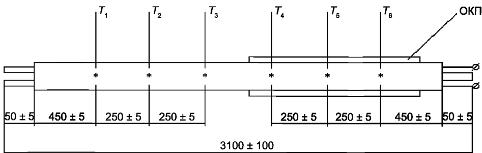
Рис. 1 — Размещение термоэлектрических преобразователей
