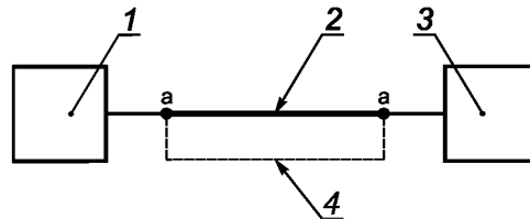
1 — генератор высокочастотных сигналов (встроенный генератор селективного микровольтметра); 2 — измерительный кабель; 3 — приемное устройство с индикатором; 4 — измеряемый фидерный тракт
