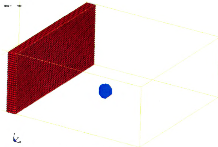
Время – 0.5 мс после взрыва
