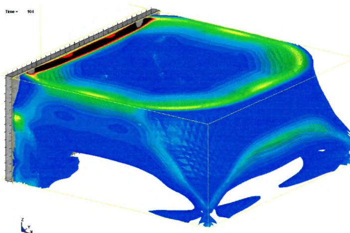
Время – 4.0 мс после взрыва
