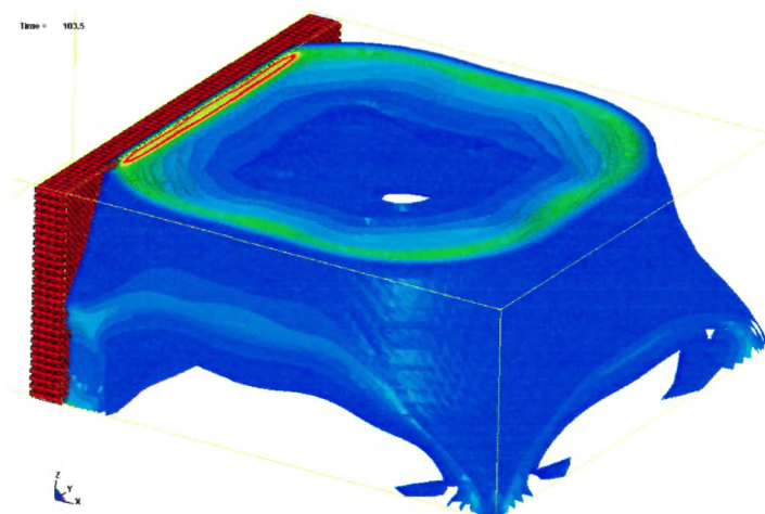
Время – 5.0 мс после взрыва
