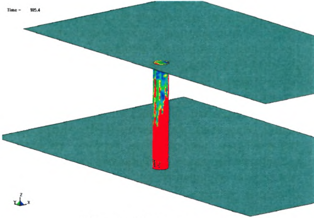
Время – 5.4 мс после взрыва
