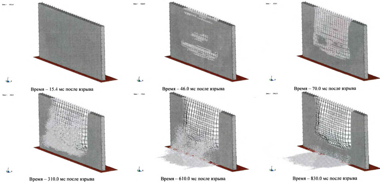
Рисунок В.25 - Фрагментация железобетонной стены при разрушении
