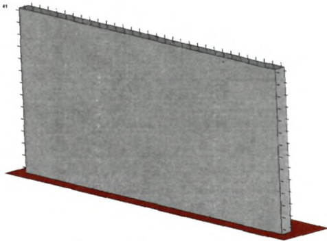
Время – 15.4 мс после взрыва
