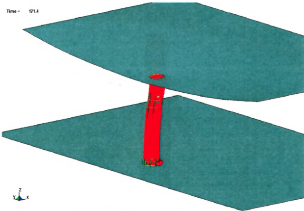
Время – 71.4 мс после взрыва
