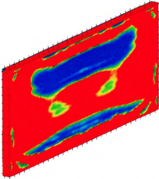
Время – 5.0 мс после взрыва
