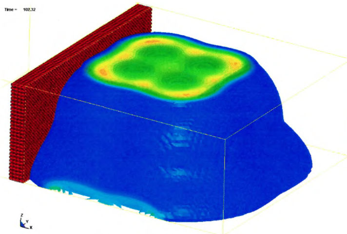
Время – 3.0 мс после взрыва
