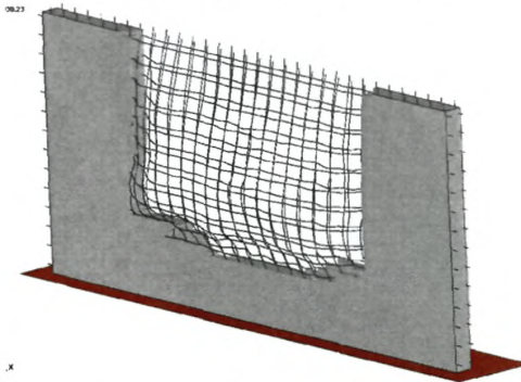
Время – 830.0 мс после взрыва
