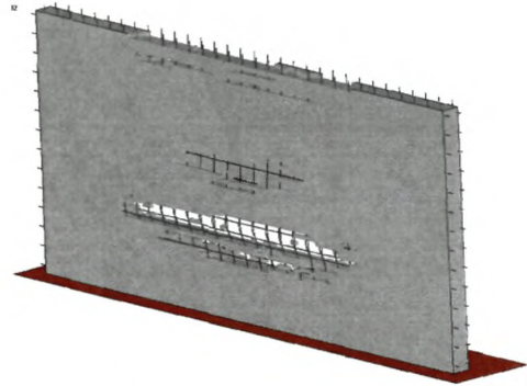
Время – 46.0 мс после взрыва
