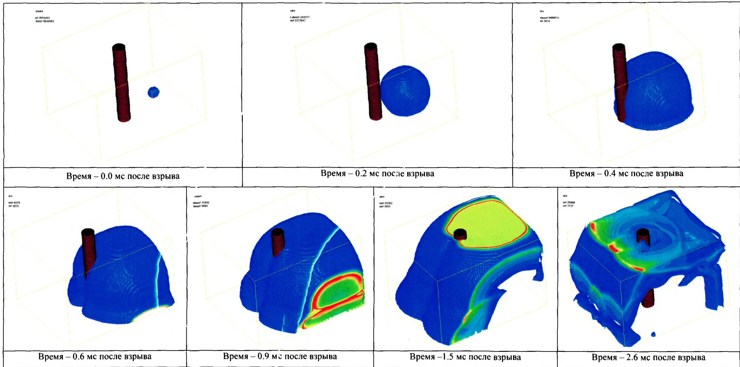
Рисунок В.4 - Обтекание колонны ударной волной
