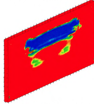
Время – 10.5 мс после взрыва
