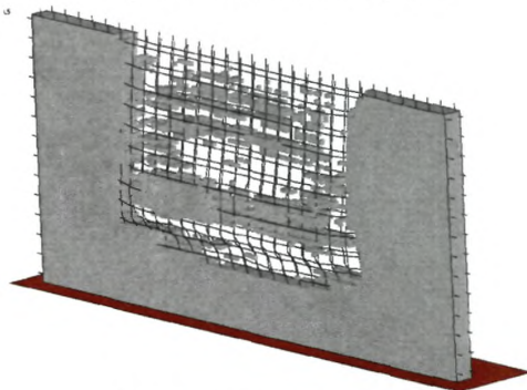
Время – 70.0 мс после взрыва
