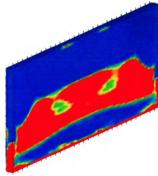
Время – 3.0 мс после взрыва
