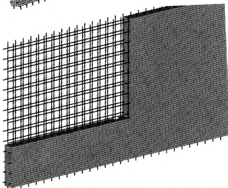
Рисунок В.15 - Геометрические и сеточные модели кирпичной и железобетонной стен (часть бетона не показана)
