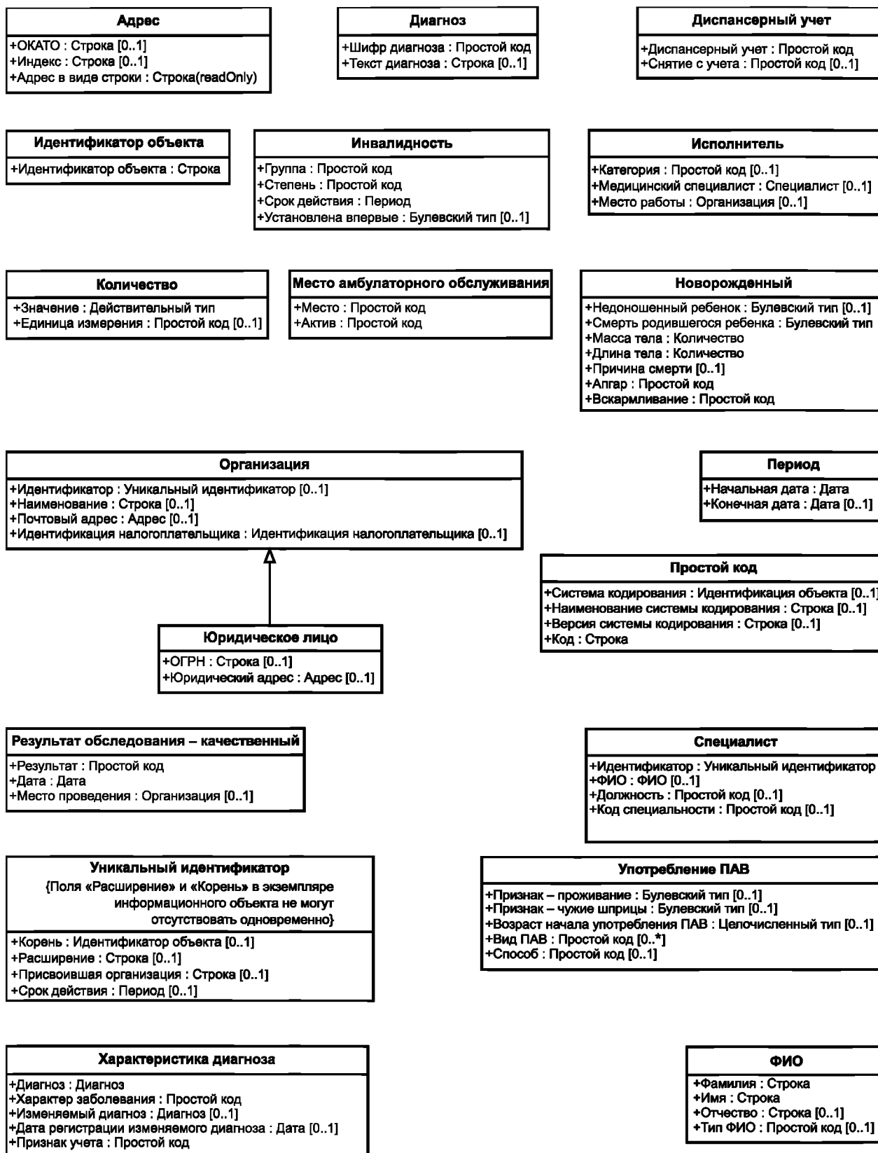
Рисунок А.4 — Вспомогательные классы
