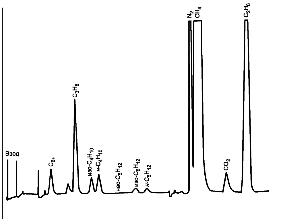
Рисунок 2 — Пример типичной хроматограммы
