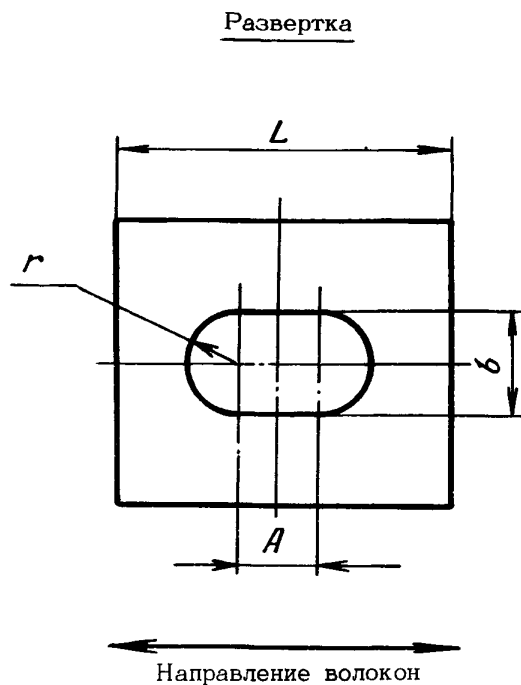
Размеры, мм
