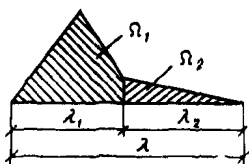
Рис. 1. Линия влияния четырехугольного очертания
