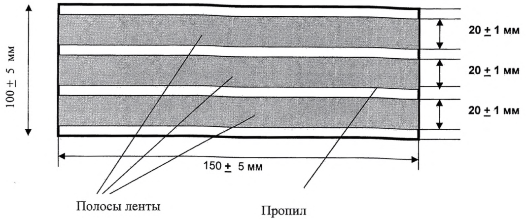
Рисунок 1 - Образец для определения адгезии покрытия при отслаивании под углом 90^{\circ} \pm 10^{\circ}
