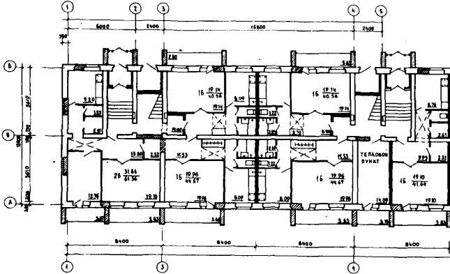
Изменение планировки типового этажа
