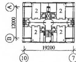
План 7-го этажа рядовой секции
