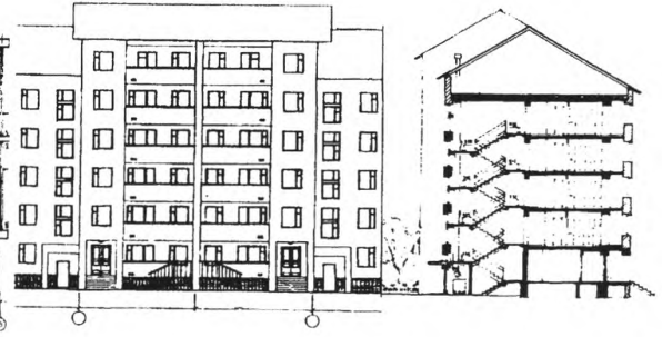
Фрагмент фасада и разрез
