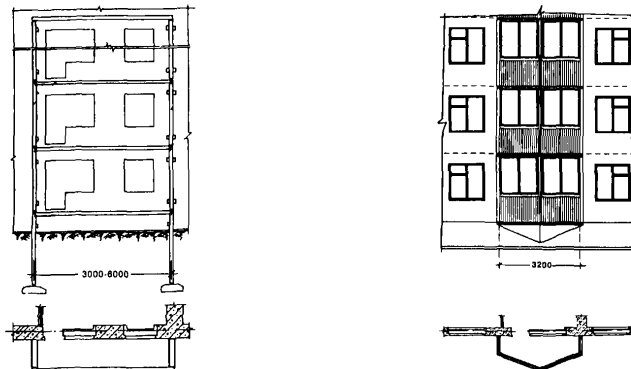
Устройство лоджий, эркеров (ризалитов)
