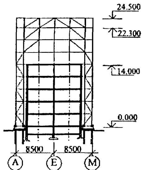
Разрез-схема
