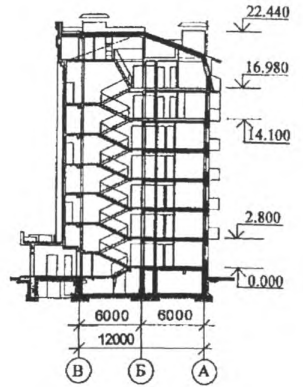
Разрез
