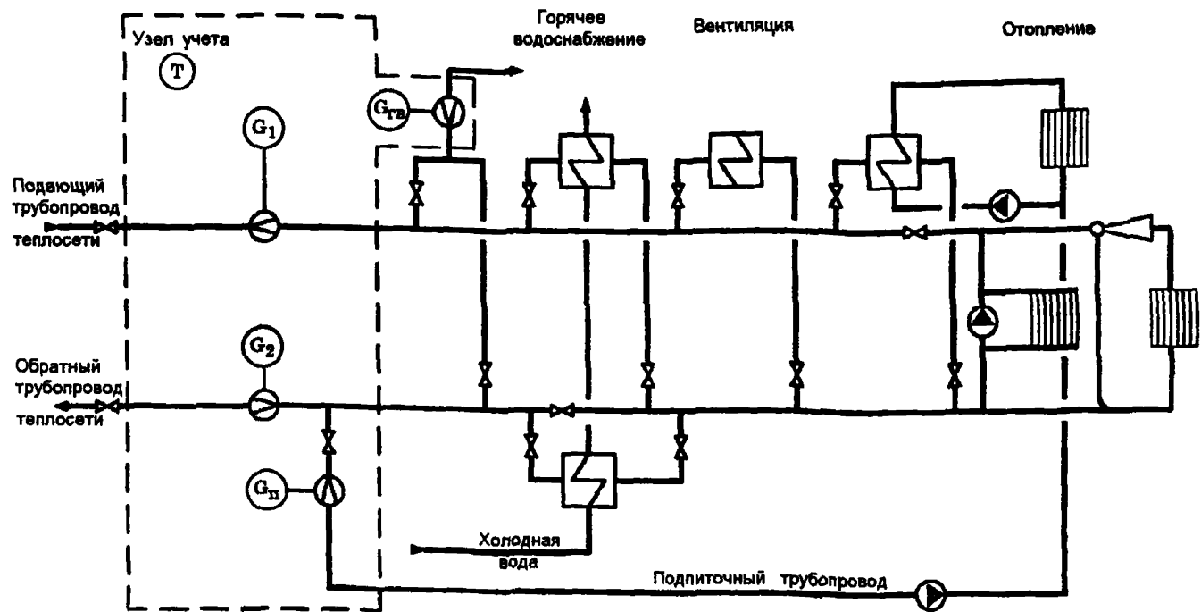
Рис 7 Принципиальная схема размещения точек измерения количества тепловой энергии и массы (объема) теплоносителя в открытых системах теплоснабжения с суммарной тепловой нагрузкой, не превышающей 0,1 Гкал/ч
