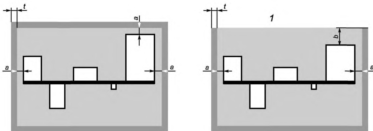
Пластмассовый корпус со всех сторон
