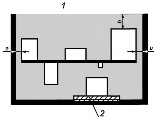
Металлический корпус не со всех сторон
