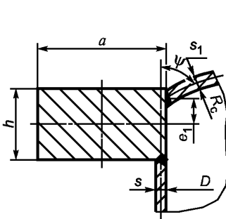
Рисунок 13 — Сферическое неотбортованное днище с укрепляющим кольцом
