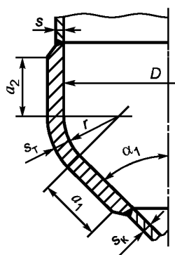
Рисунок 26 — Соединение обечаек с тороидальным переходом
