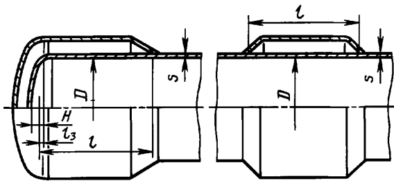
Рисунок 3 — Гладкие обечайки с рубашкой
