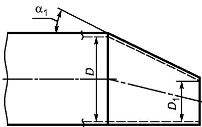
Рисунок 28 — Соединение кососимметричных обечаек
