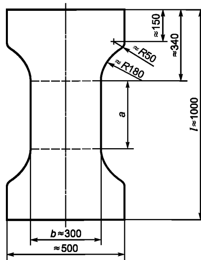
Рисунок 2 — Форма и размеры испытуемого образца
