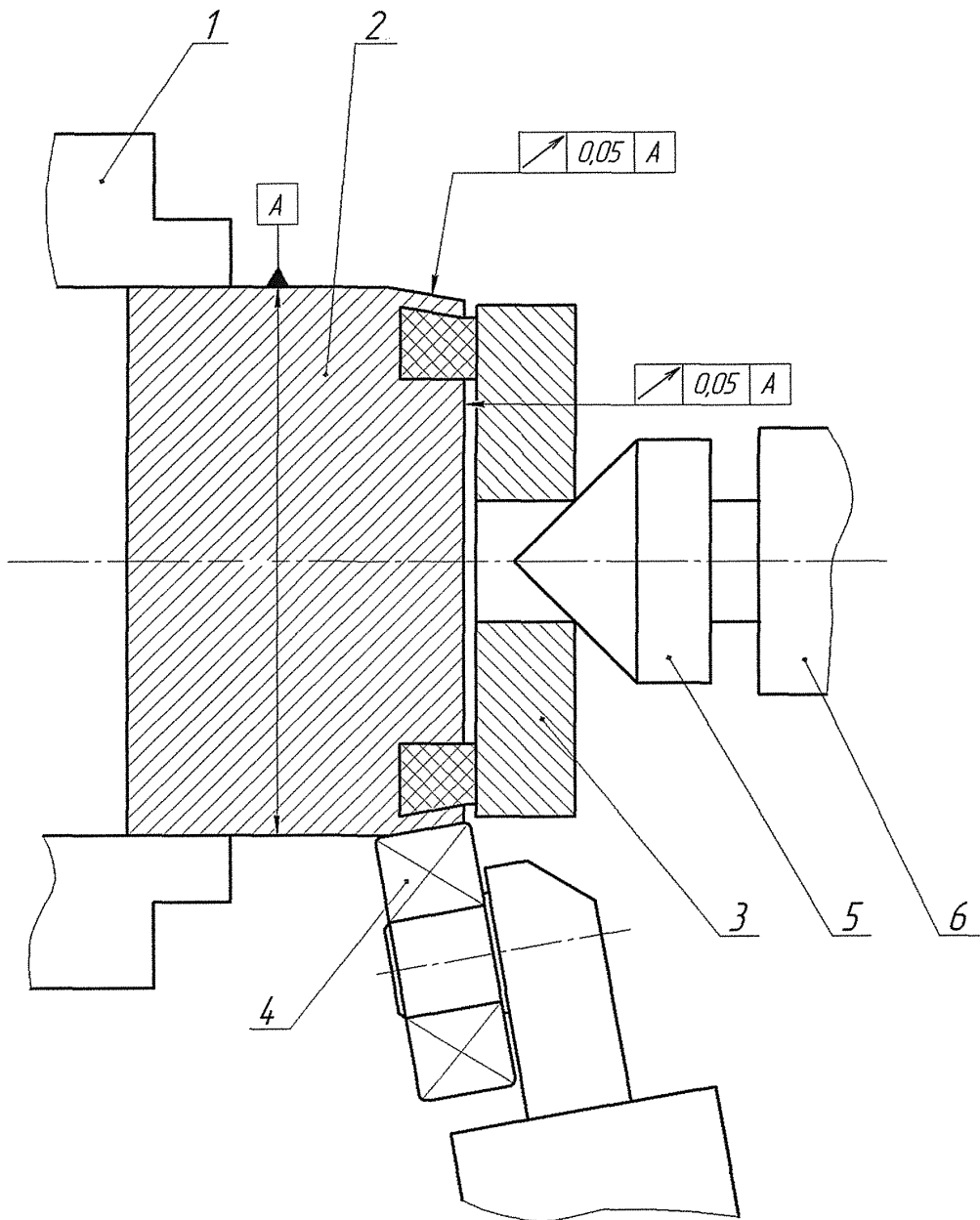
1 – шпиндель; 2 – золотник; 3 – прижимы; 4 – ролик; 5 – вращающийся центр; 6 – скалка; 7 – резцедержатель.
