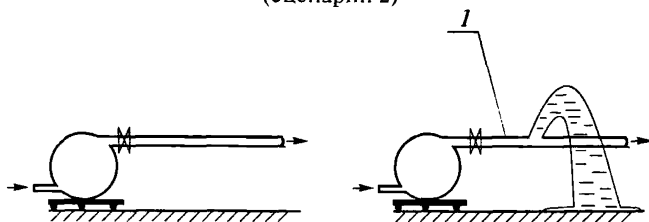
Рис. 4.10. Разгерметизация трубопровода с жидкой фазой, присоединенного к насосу ( I — отсекаемый участок аварийного трубопровода) (сценарий 4)
