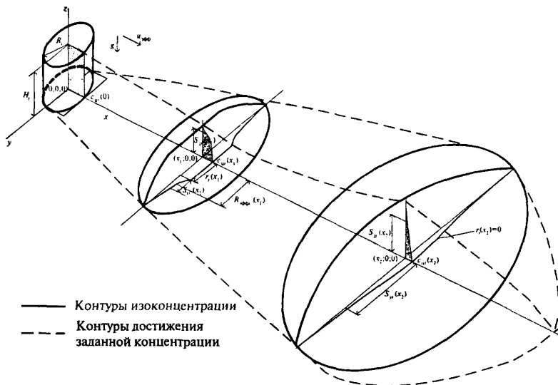
Рис. 3.1. Схема распространения первичного облака
