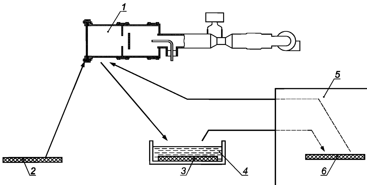
1 — устройства для измерения эффективности; 2 — образец фильтрующего материала; 3 — обработка изопропанолом; 4 — кювета (емкость) с изопропанолом; 5 — вытяжной шкаф; 6 — сушка образца материала
