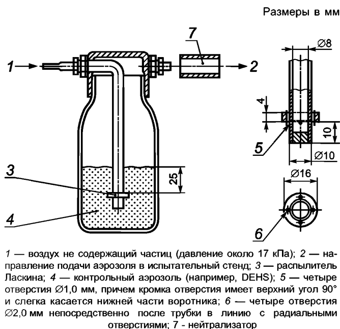
Рисунок 4 — Система генерирования частиц DEHS
