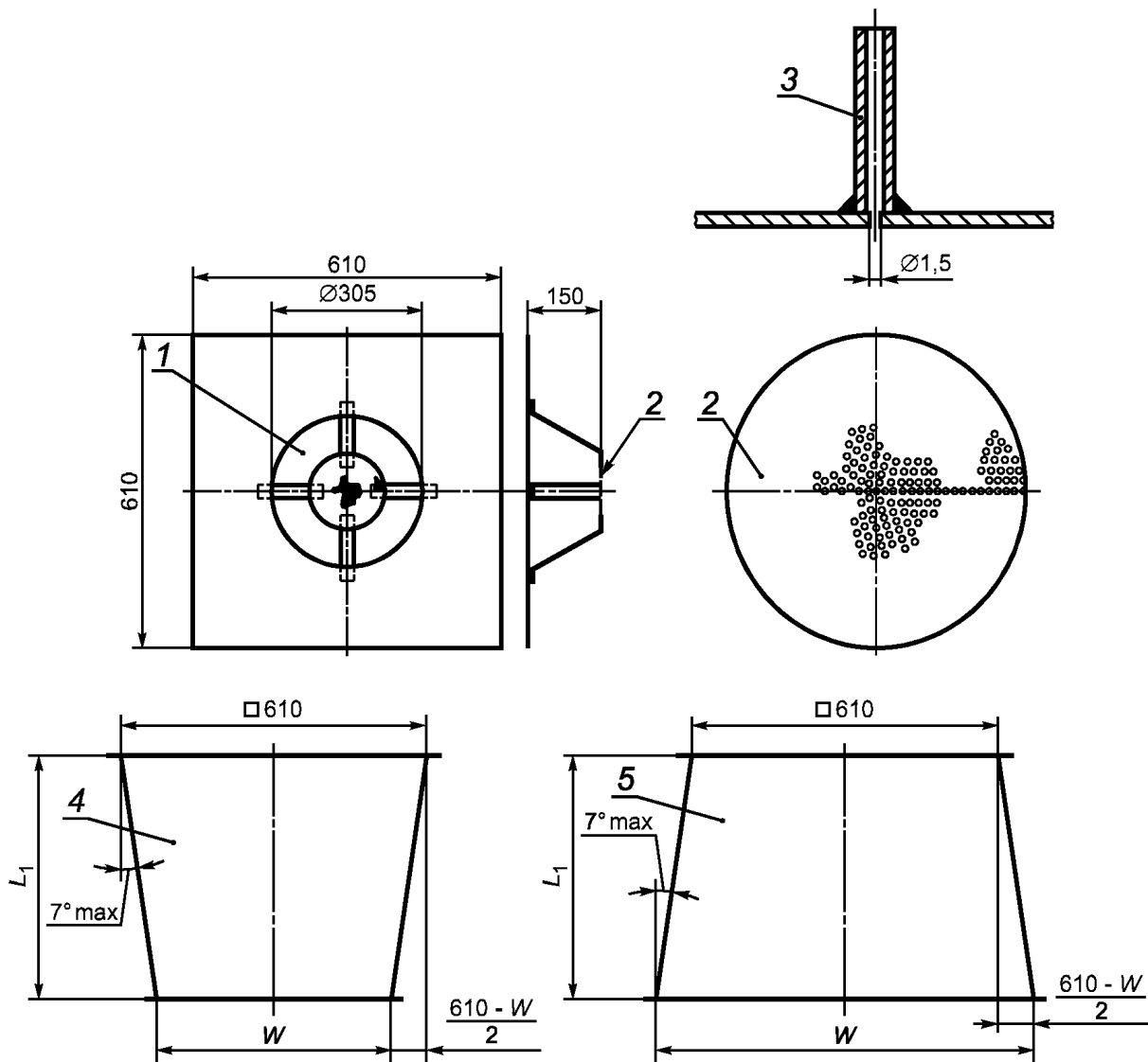
1 — смешивающее отверстие; 2 — перфорированная пластина Ж152 ± 2 мм, отверстия занимают 40 % площади; 3 — отвод для измерения давления; 4 — переходной элемент воздуховода (фильтр меньше сечения воздуховода); 5 — переходной элемент воздуховода (фильтр больше сечения воздуховода)
