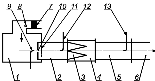
Рисунок 1 — Схема испытательного стенда
