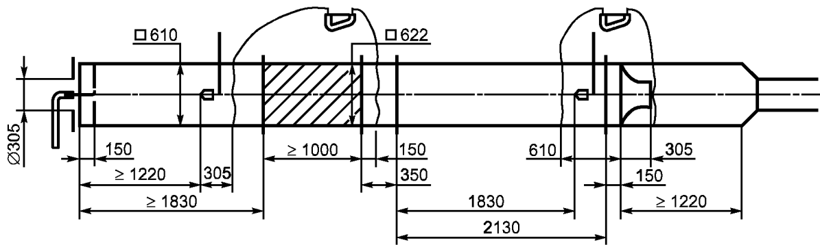
Рисунок 2 — Размеры испытательного стенда
