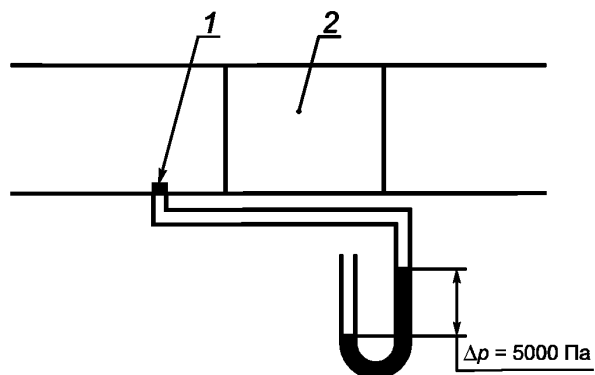
1 — закрытое отверстие отбора давления; 2 — секция испытательного устройства
