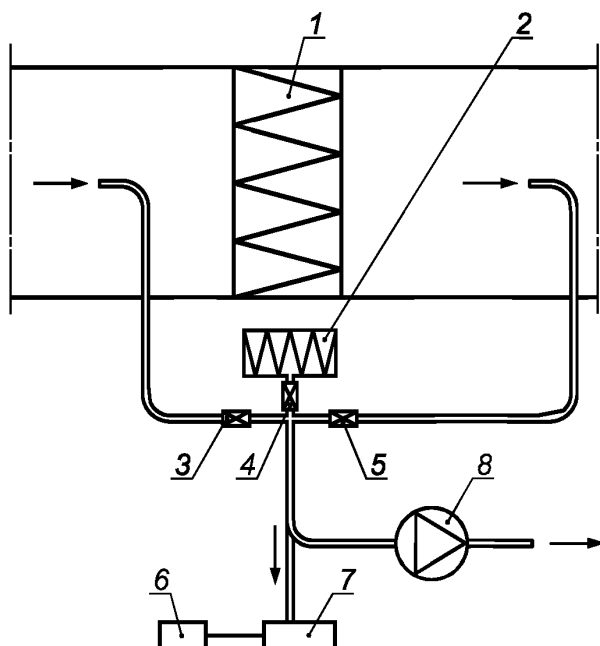
1 — фильтр; 2 — HEPA-фильтр (чистый воздух); 3 — клапан до фильтра; 4 — клапан чистого воздуха; 5 — клапан после фильтра; 6 — компьютер; 7 — счетчик частиц; 8 — насос
