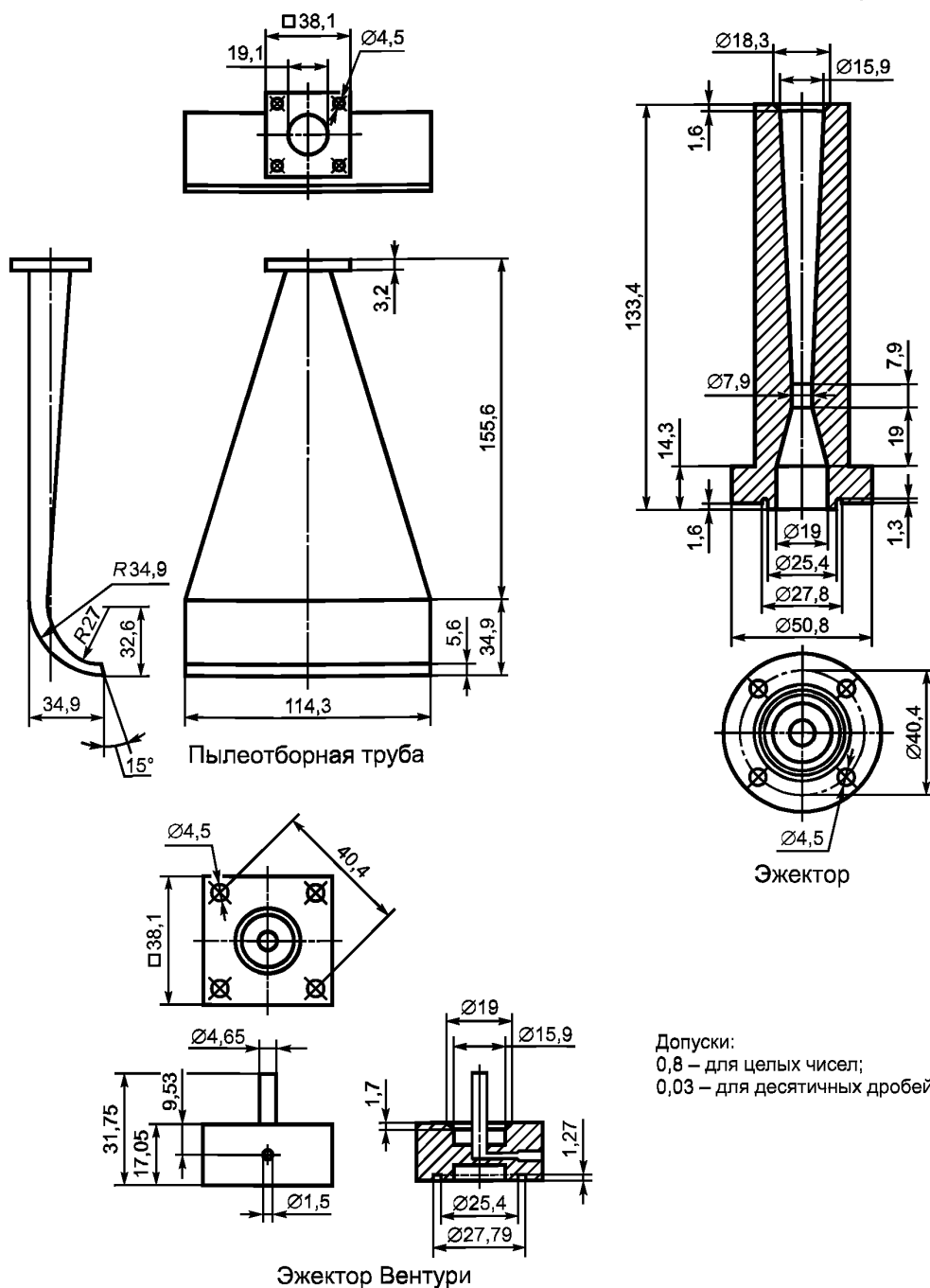
Рисунок 7 — Эжектор, эжектор Вентури и детали линии подачи пыли
