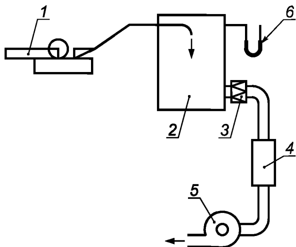
Рисунок 10 — Схема определения расхода воздуха генератора пыли
