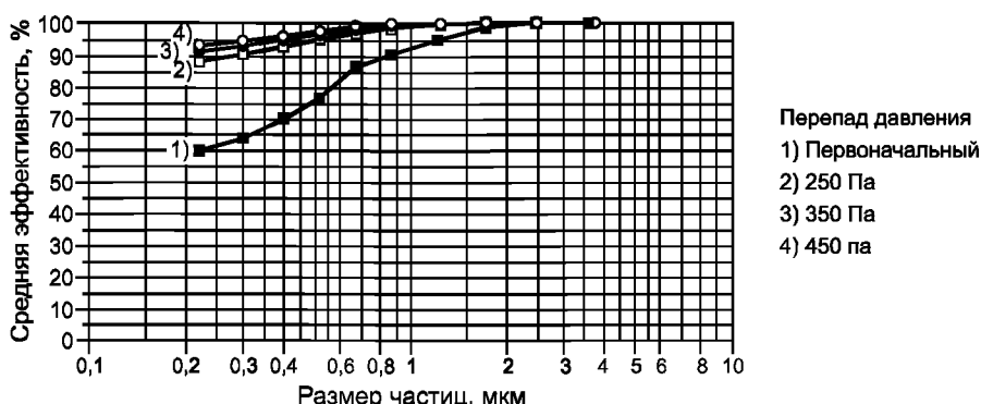
Рисунок Е.3 — Начальная и средняя эффективность при различных конечных перепадах давления
