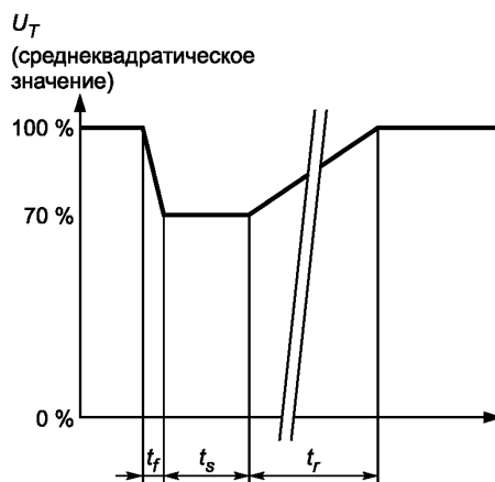
Рисунок 3 — Изменение напряжения
