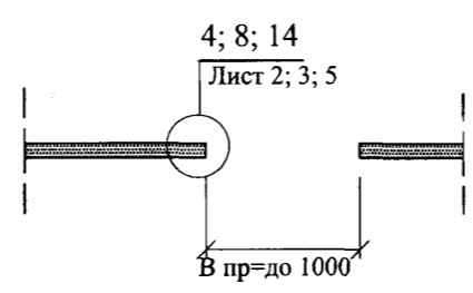
1 - 1 при двойных ( межквартирных ) перегородках
