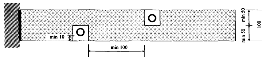
Рис. 6. Монтаж трубопроводов небольшого диаметра в одинарной перегородке
