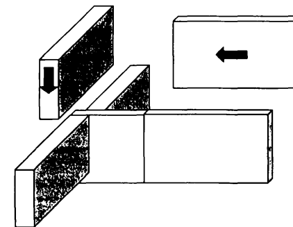
Рис. 4. Монтаж плит при пересечении перегородок друг с другом
