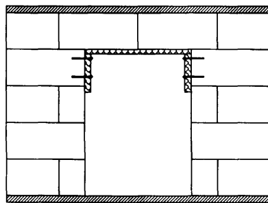
Рис. 3. Монтажная конструкция при устройстве дверного проема
