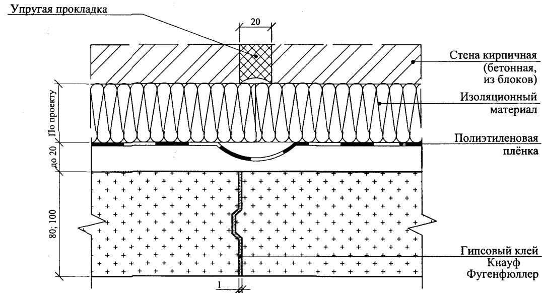
Температурный шов
