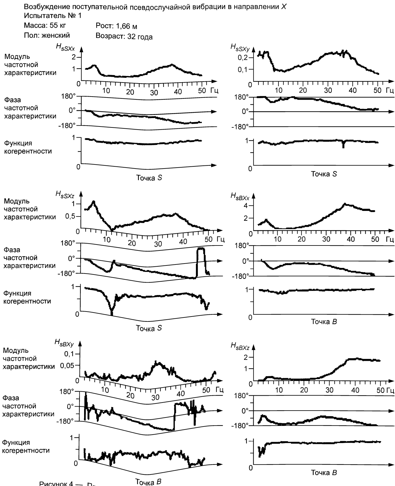
Рисунок 4 — Пример результатов испытания с возбуждением псевдослучайной вибрации
