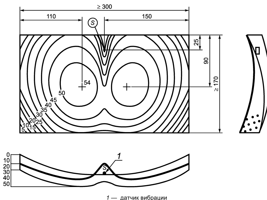
Рисунок 3 — Чашка сиденья (чертеж)
