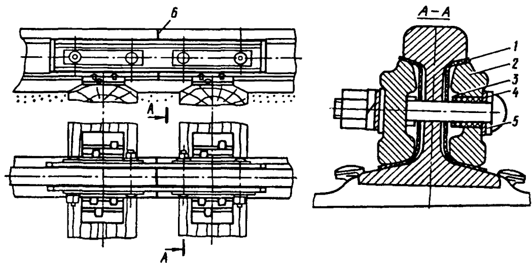
Рис. 339. Изолирующий стык с двухголовыми металлическими накладками для пути с деревянными шпалами: 1 — боковая прокладка; 2 — накладка; 3 — втулка; 4 — изолирующая планка под болт; 5 — стопорная планка; 6 — торцовая прокладка
