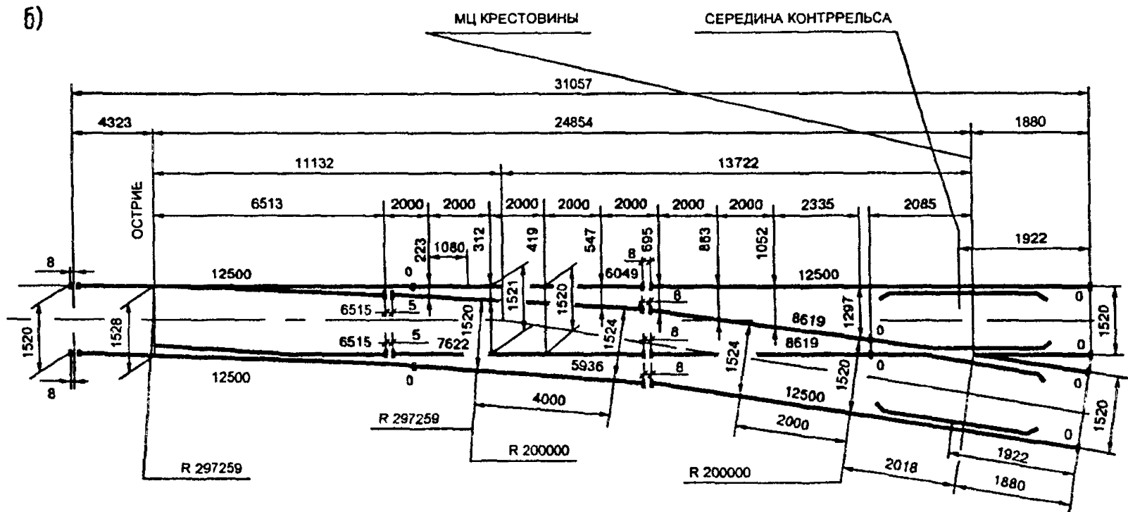
Рис. 5.24. Эпюра укладки (а) и схема разбивки (б) стрелочного перевода типа Р50 марки 1/9. Проект 2643
