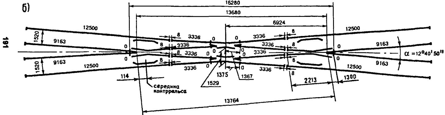
Рис. 5.21. Эпюра укладки (а) и схема разбивки (б) глухого пересечения типа Р65 марки 2/9. Проект 1684
