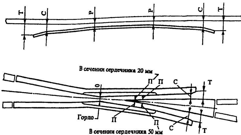
Рис. 3.12. Места контрольных измерений ширины желобов в острых крестовинах и в контррельсах
