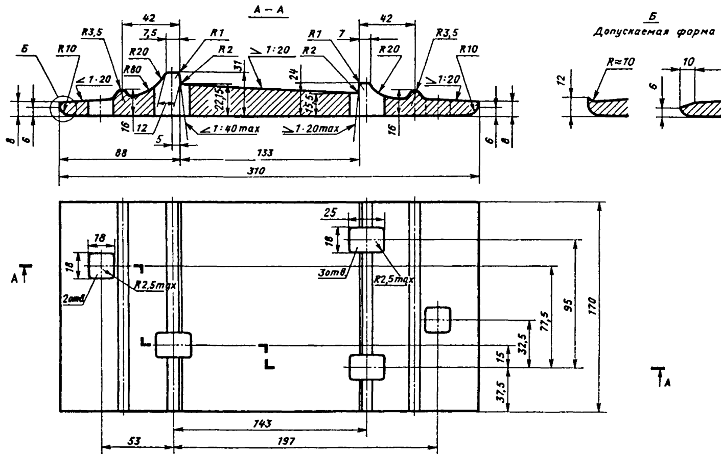
Рис. П.2.8. Подкладка Д50 костыльного скрепления к рельсам типа Р50
