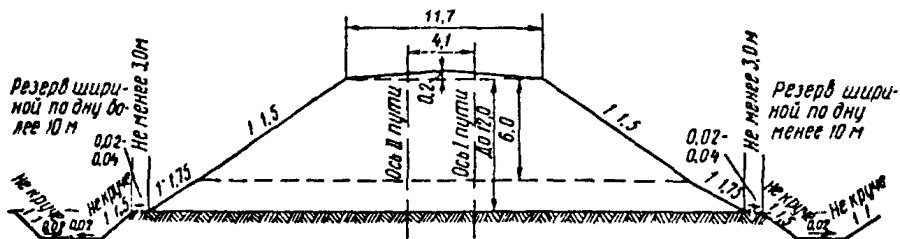
Рис. П.6.3. Насыпь высотой до 12 м с шириной основной площадки 11,7 м при поперечном уклоне местности не круче 1:5
