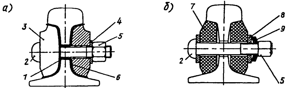
Рис. 3.41. Изолирующий стык: а — клеebolтовой с металлокомпозитными накладками; б — сборный с композитными накладками из стеклопластика; 1 — изолирующий слой; 2 — стыковой болт; 3 — металлокомпозитная накладка; 4 — изолирующая втулка; 5 — гайка; 6 — боковая изоляция; 7 — композитная накладка из стеклопластика; 8 — стопорная планка; 9 — тарельчатая пружина (пружинная шайба)
