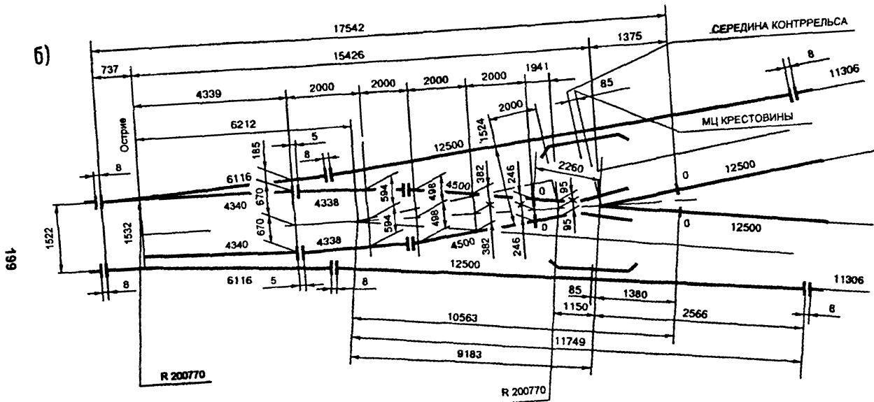
Рис. 5.25. Эпюра укладки (а) и схема разбивки (б) симметричного стрелочного перевода типа Р50 марки 1/6 для горочных путей. Проект 1581
