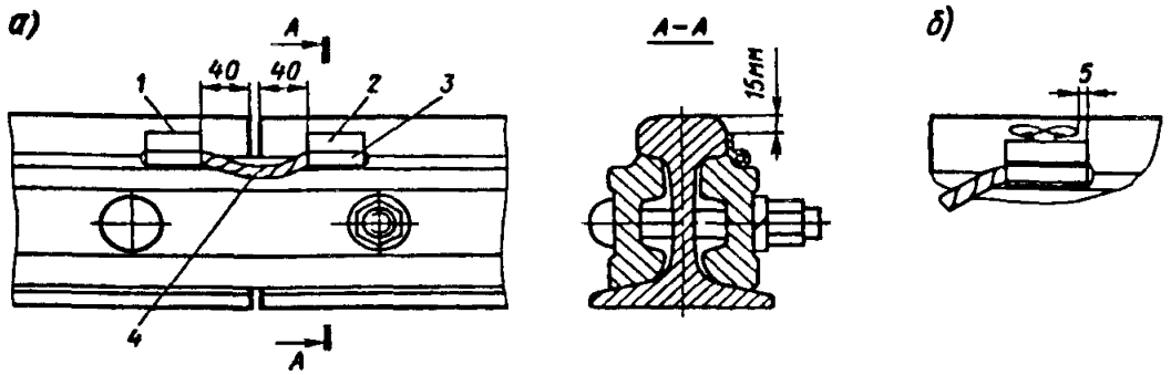
Рис. 3.34. Схема установки (а) и приварки (б) медного соединителя фартучного типа к головке рельса: 1 — шов, выполняемый ручной электродугуговой сваркой, 2 — фартук; 3 — наконечник (манжета); 4 — гибкий трос МГГ-70
