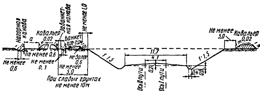
Рис. П.6.4. Выемка глубиной до 12 м с шириной основной площадки 11,7 м при поперечном уклоне местности не круче 1:3
