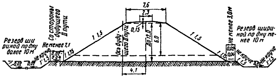
Рис. П.6.1. Насыпь высотой до 12 м с шириной основной площадки 7,6 м при поперечном уклоне местности не круче 1:5
