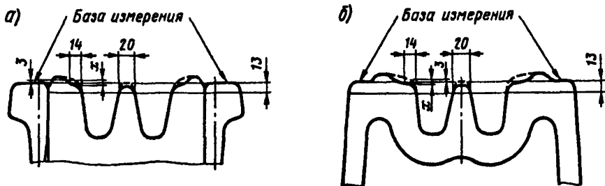
Рис. 3.19. Измерение вертикального износа x усювиков сборной (а) и цельнолитой (б) острых крестовин
