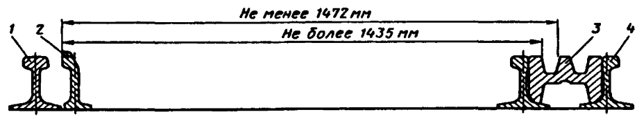
Рис. 3.23. Схема измерения расстояний между рабочими гранями контррельса и усювика и рабочими гранями контррельса и сердечника крестовины: 1 — путевоу рельс; 2 — контррельс; 3 — сердечник; 4 — усювик
