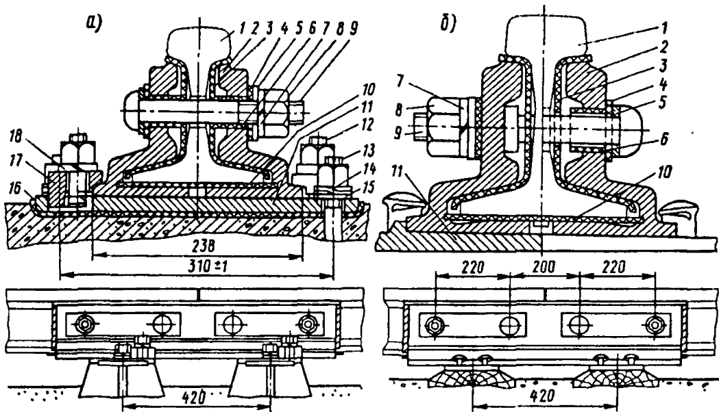
Рис. 338. Изолирующий стык с объемлющими металлическими накладками: a — при железобетонных шпалах и скреплении КБ; б — при деревянных шпалах с костыльным скреплением; 1 — рельс; 2 — накладка; 3 — прокладка боковая; 4 — полиэтиленовая планка под болты; 5 — металлическая стопорная планка; 6 — втулка; 7 — пружинная шайба; 8 — гайка; 9 — стыковой болт; 10 — изолирующая прокладка под рельс; 11 — подкладка; 12 — клеммный болт; 13 — закладной болт; 14 — пружинная шайба; 15 — плоская шайба; 16 — прокладка под подкладку; 17 — клемма; 18 — шайба
