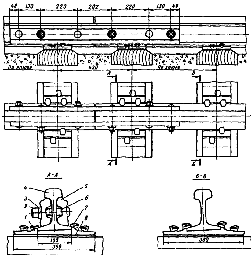
Рис. 3.1. Стыковое и промежуточное крестовое скрепление при рельсах Р65, Р75: 1 — подкладка Д65; 2 — гайка М27; 3 — пружинная одновитковая шайба; 4 — рельс типа Р65; — двухголовая накладка; 6 — путевой болт М27×160; 7 — путевой костыль; 8 — прокладка под подкладку
