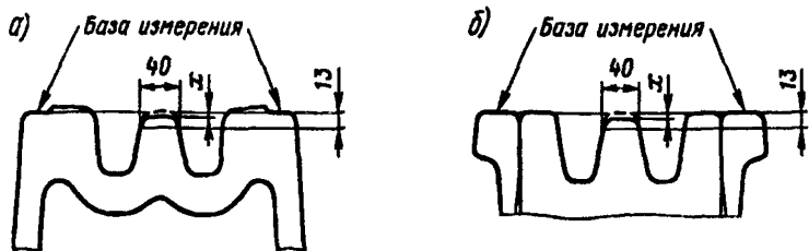
Рис. 3.17. Измерение вертикального износа x сердечника цельнолитой (а) и сборной (б) крестовин
