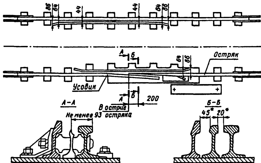
Рис. 3.29. Башмакосбрасыватели типов Р50, Р65 колес 1520 мм: * — на расстоянии 200 мм от острия острья и до конца усовика
