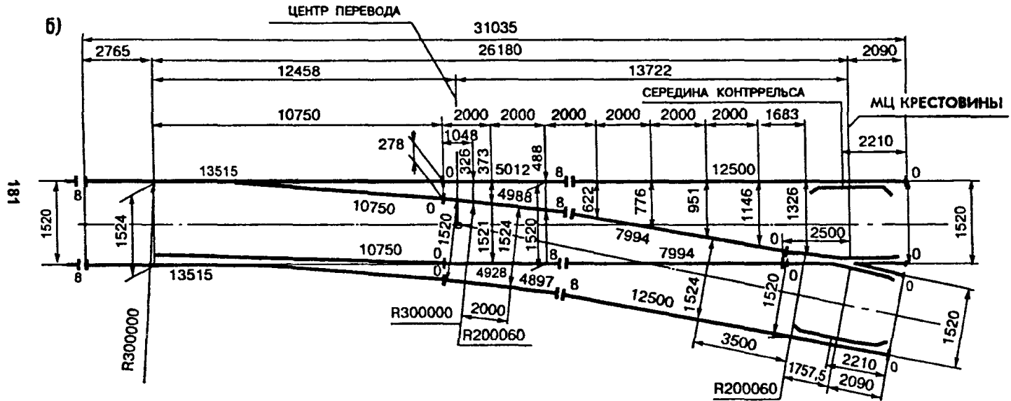
Рис. 5.16. Эпюра укладки (а) и схема разбивки (б) стрелочного перевода типа Р65 марки 1/9. Проект 2721
