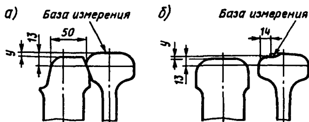
Рис. 3.25. Измерение понижения остряка относительно рамного рельса у при равномерном (а) и неравномерном (б) вертикальном износе рамного рельса
