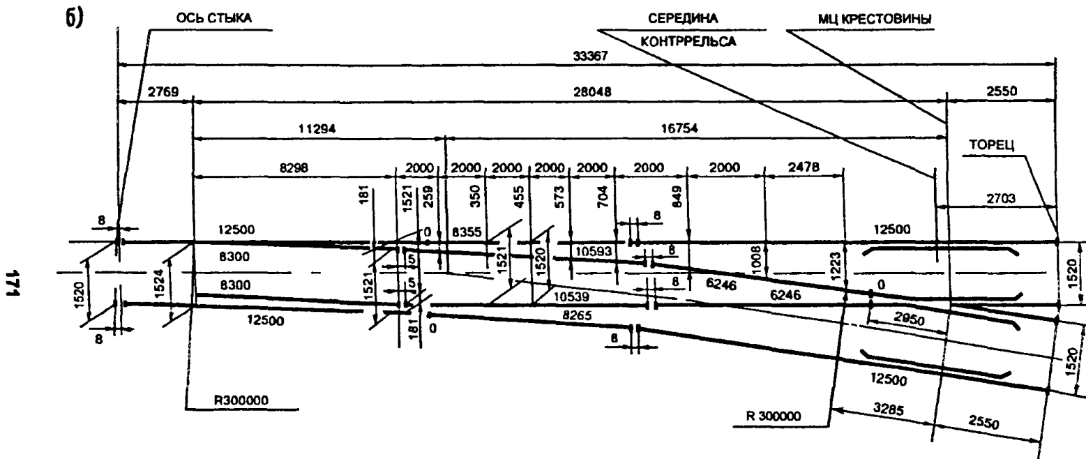
Рис. 5.11. Эпюра укладки (а) и схема разбивки (б) стрелочного перевода типа Р65 марки 1/11 на железобетонных брусках. Проекты 2768 и 1740
