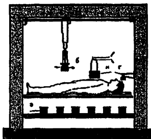
Рис. 5.1. СИЧ экспертного класса, геометрия измерения "лежа"
