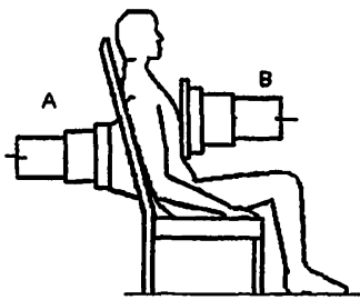
Рис. 5.3. СИЧ оперативного класса, геометрия "измерительное кресло"
