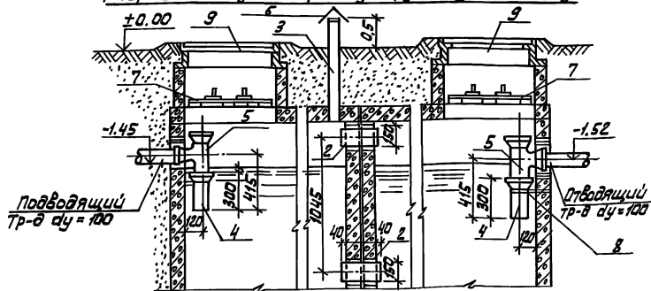
Разрез по двухкамерному круглому септику
