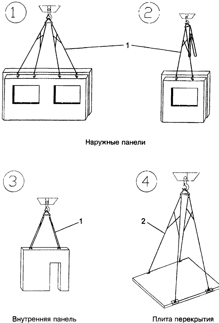
Рис. 1. Схемы строповки
