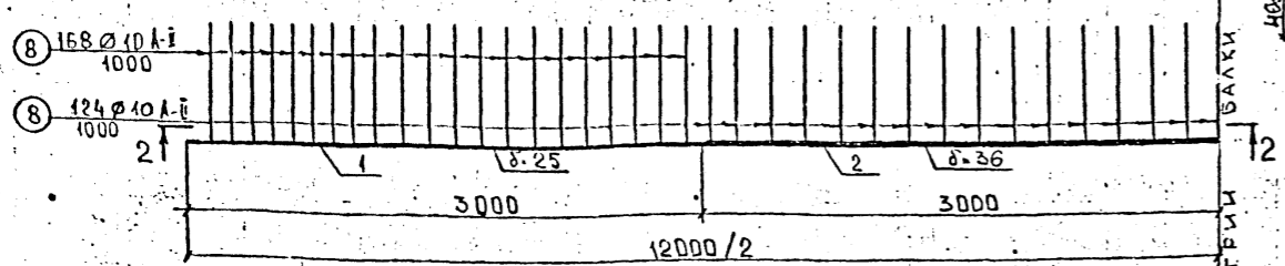
Расположение хомутов на листе внешнего армирования балки
