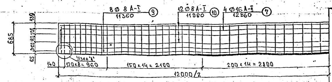
Расположение хомутов на листе внешнего армирования балки
