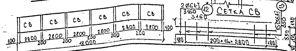
ПЛАН СЕТОК ВУТОВ
