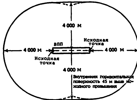
Рис. 1-1. Внутренняя горизонтальная поверхность для одной ВПП (кодový номер ВПП - 4)
