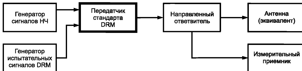
Рисунок 34 — Структурная схема измерений параметров передатчика DRM
