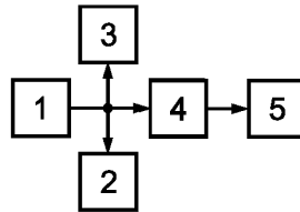
1 — генератор НЧ сигналов; 2 — селективный вольтметр; 3 — частотомер; 4 — канал звукового вещания; 5 — анализатор спектра или селективный вольтметр
