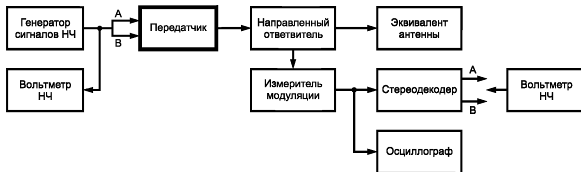
Рисунок 29 — Схема измерения неравномерности АЧХ в режиме СТЕРЕО
