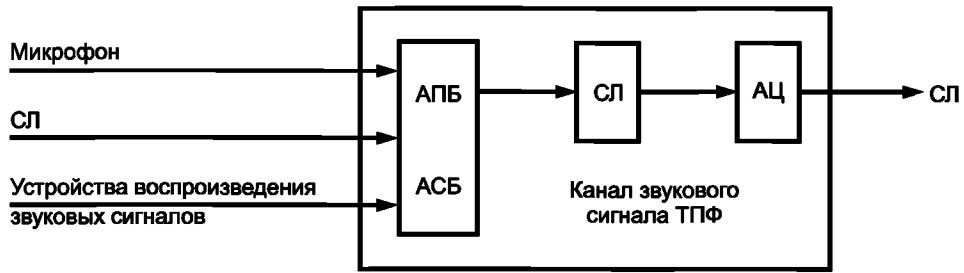
Рисунок 2 — Тракт формирования программ
