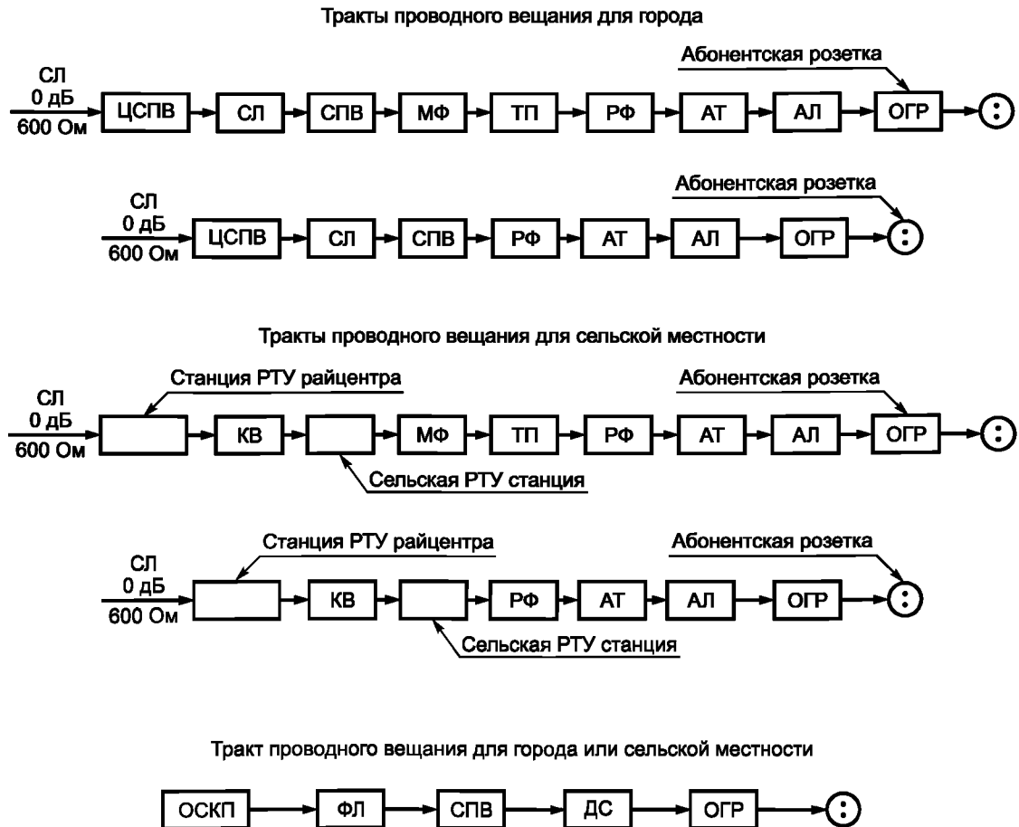
Рисунок А.1 — Структуры трактов проводного вещания
