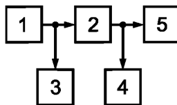
1 — низкочастотный генератор сигналов; 2 — измеряемый тракт или звено; 3, 4 — вольтметры; 5 — номинальное сопротивление нагрузки — резистор
