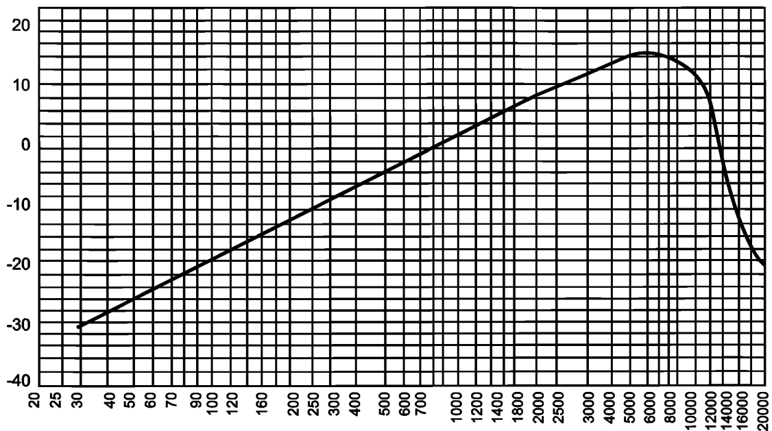
Рисунок 19 — График АЧХ псофометрического фильтра в соответствии с [1]
