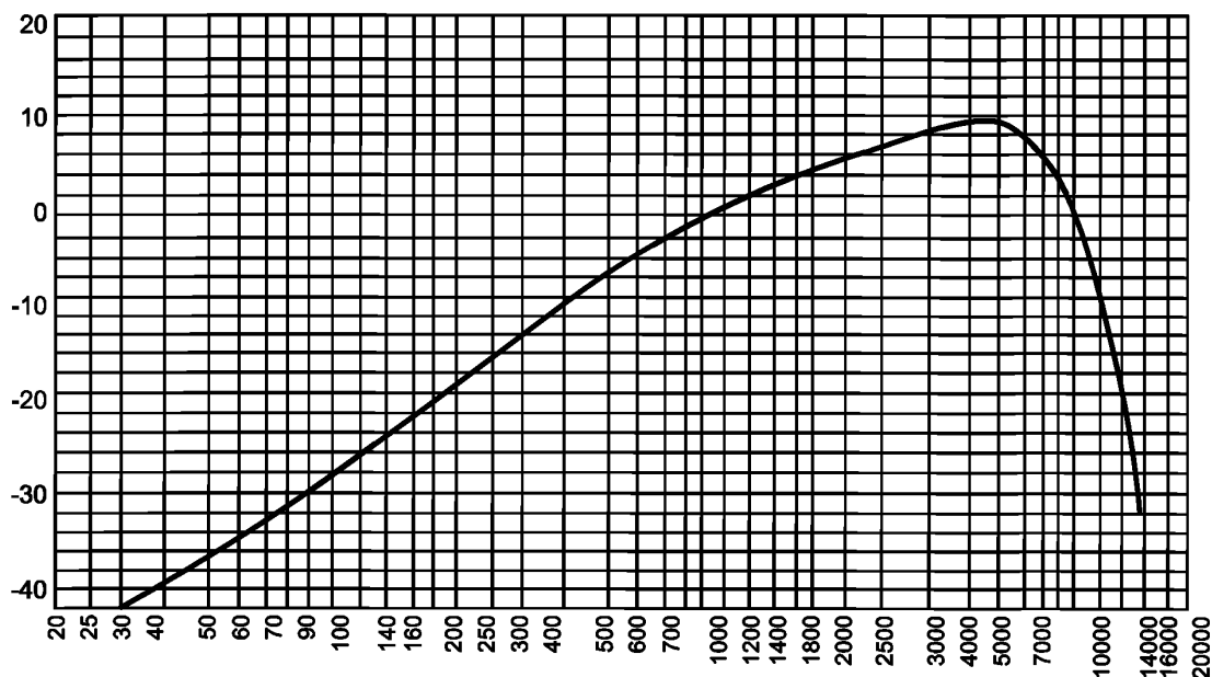
Рисунок 20 — График АЧХ псофометрического фильтра в соответствии с [6]
