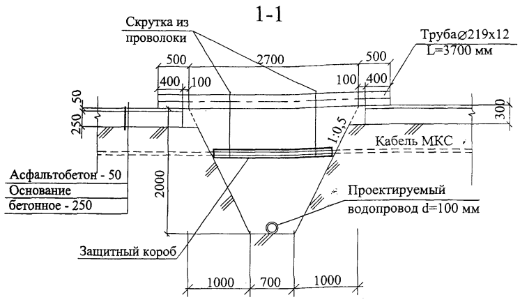
Рисунок 2- Габаритные размеры котлована.
