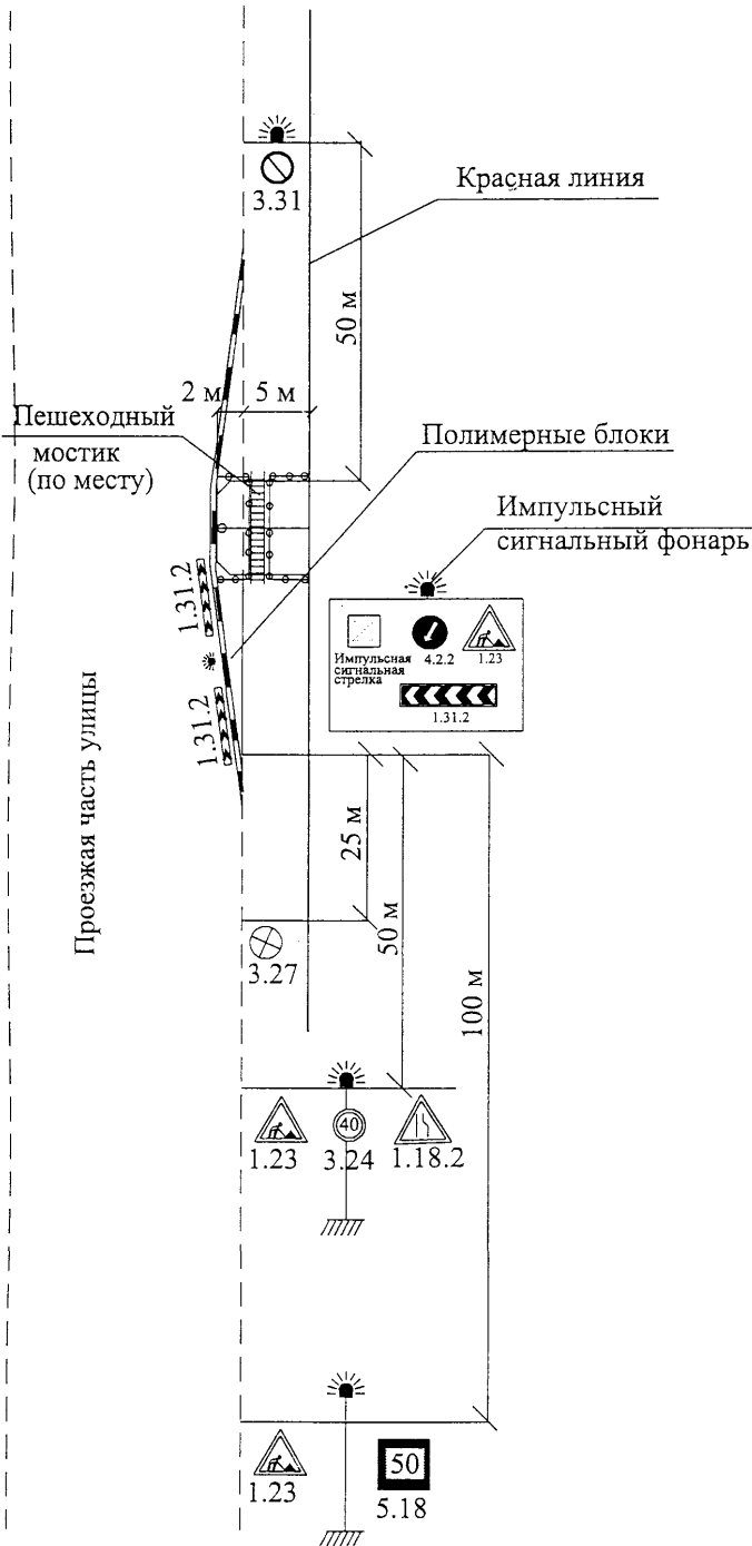
Рисунок 3- Схема организации движения.
