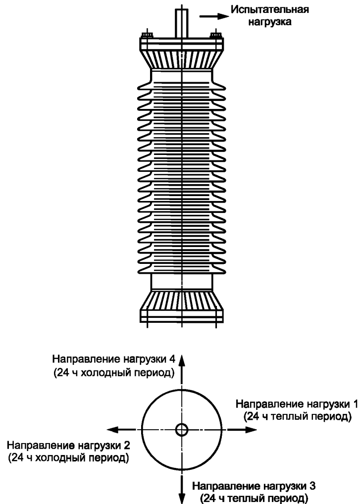
Рисунок 5 — Направления действия изгибающей нагрузки при термомеханических испытаниях
